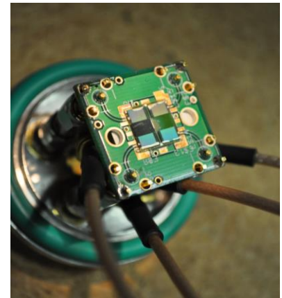
Figure 1 : capteur SAW (ligne à retard)
